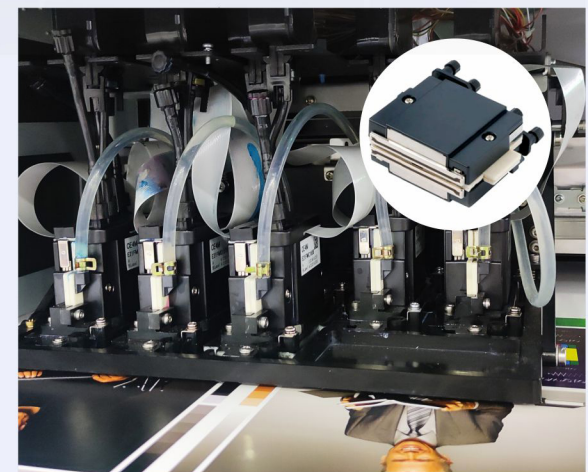
配置5个东芝CE4M工业打印头 2400dpi高清打印，画质细腻
